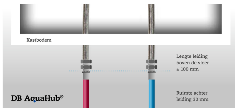
Puntstuk warmwater 1/2" bu.dr t.b.v. AquaHub
